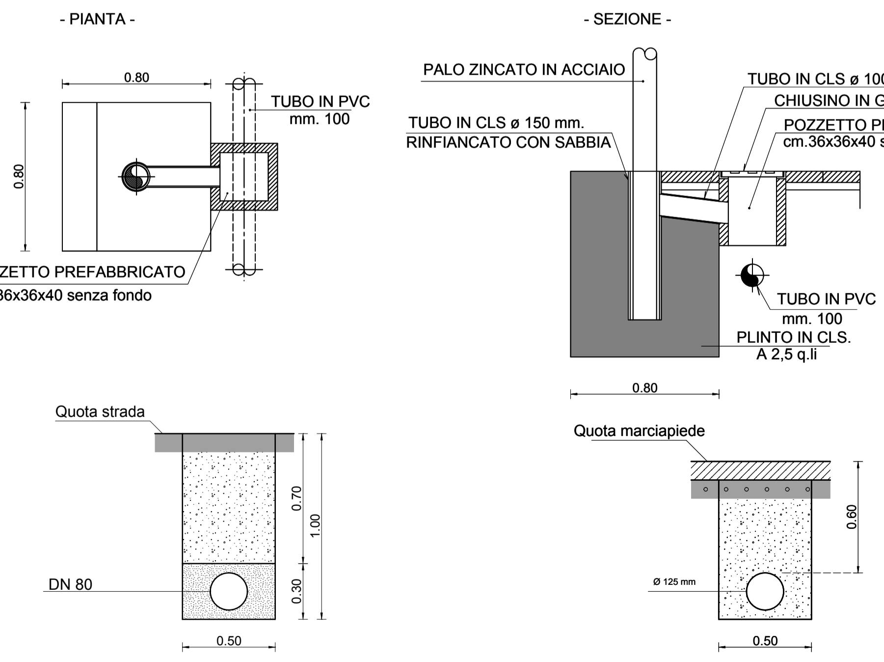
BASAMENTO TIPICO PALO CON POZZETTO D'ALLACCIO 1:20
