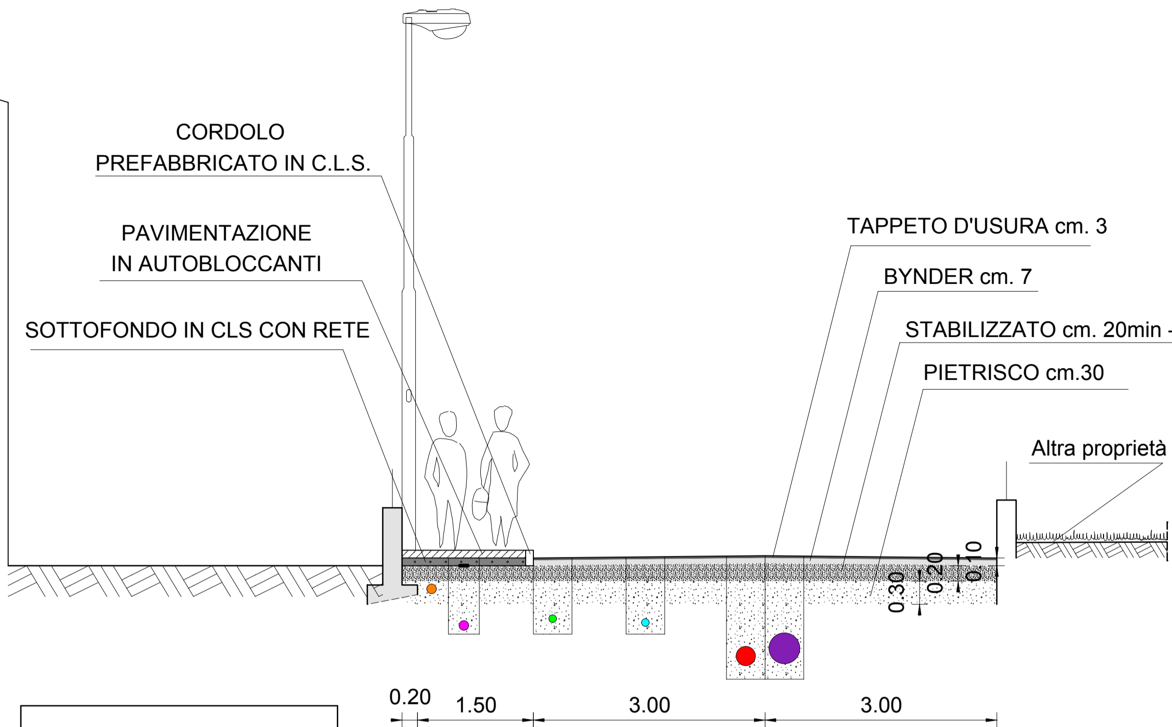
SEZIONE STRADALE SCALA 1:50
