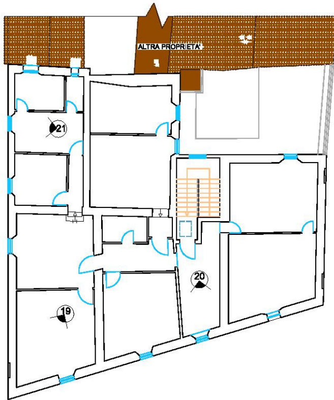
PIANO SECONDO
